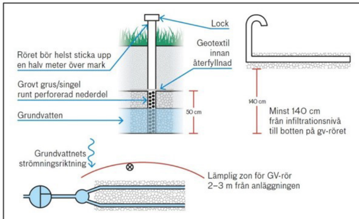
Figur 1. Detaljritning, permanent kontrollpunkt för grundvatten vid infiltration
